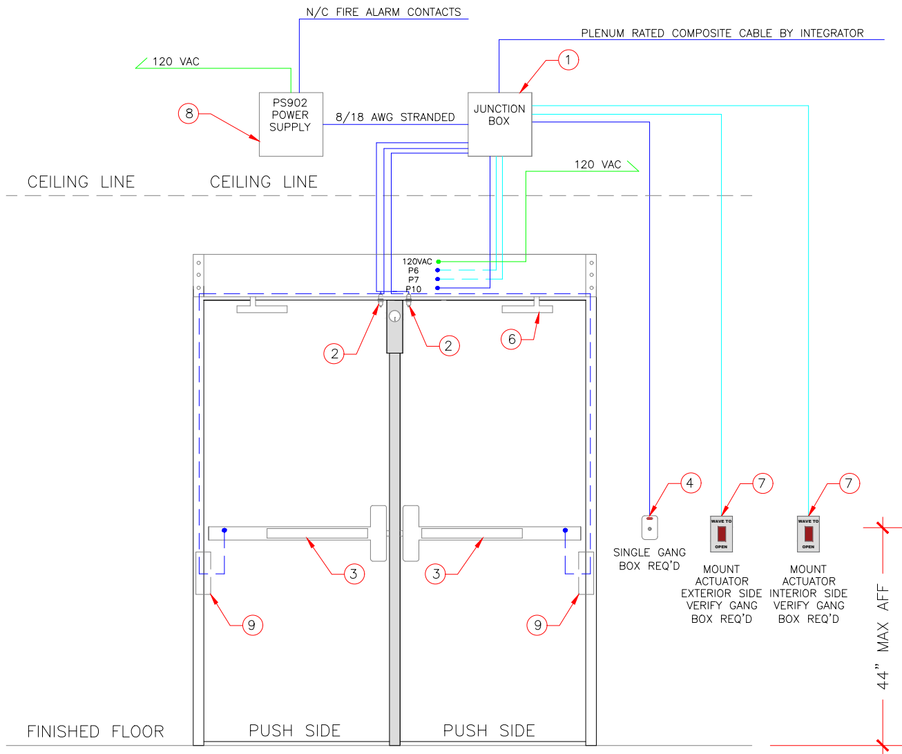
DOOR ELEVATION N.T.S.
