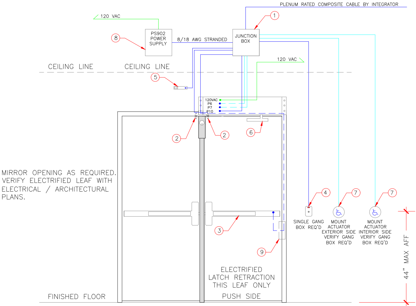
DOOR ELEVATION N.T.S.
