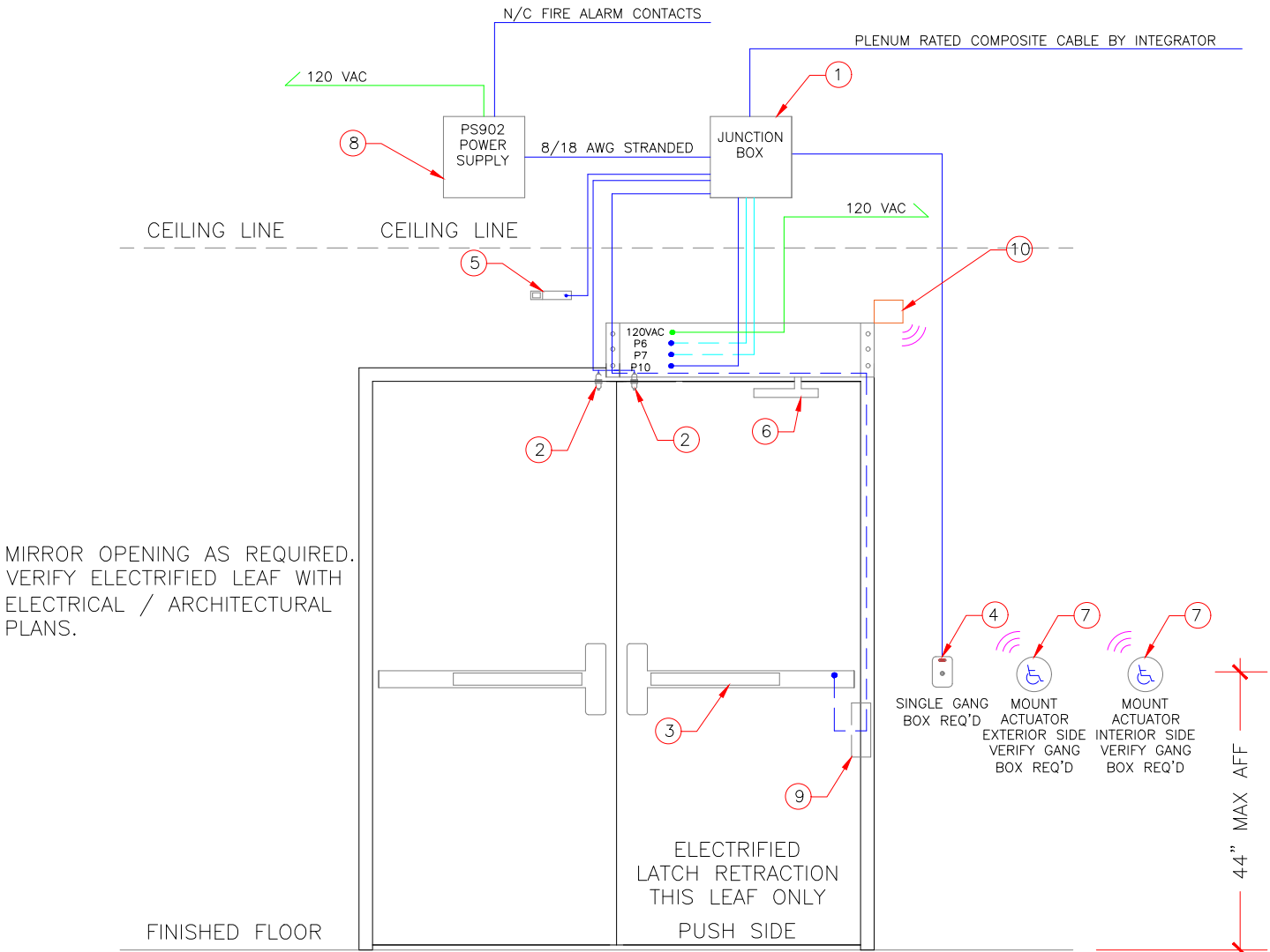
DOOR ELEVATION N.T.S.
